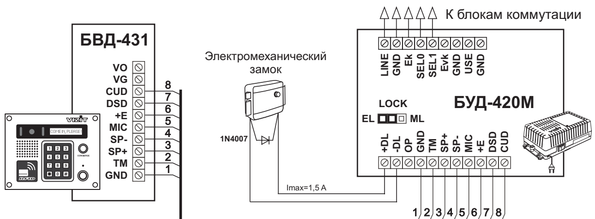
Рисунок 5 - Схема соединений блока вызова БВД-431 с блоком управления БUD-420M и электромеханическим замком
