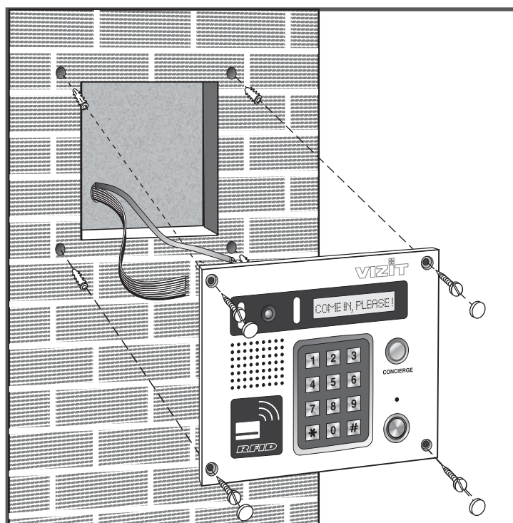
Рисунок 2 - Крепление блока вызова
