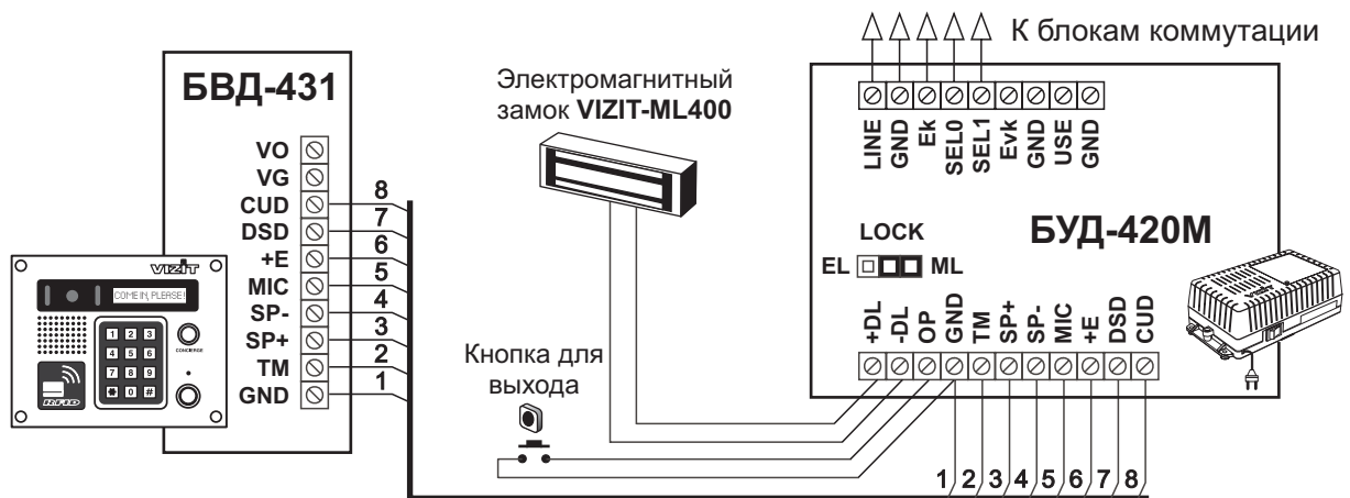
Рисунок 4 - Схема соединений блока вызова БВД-431 с блоком управления БUD-420M , электромагнитным замком VIZIT-ML400 и кнопкой для выхода
