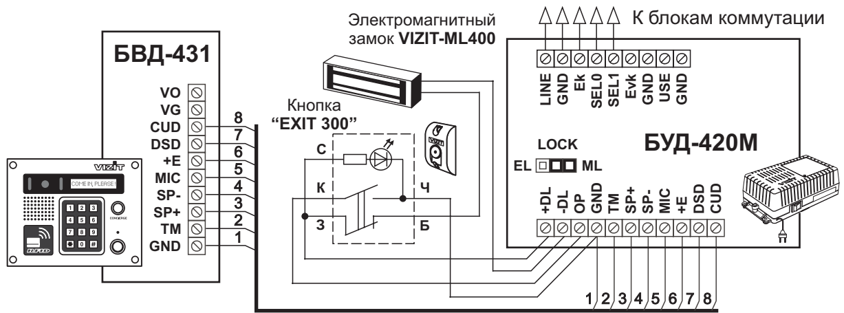
Рисунок 3 - Схема соединений блока вызова БВД-431 с блоком управления БUD-420M , электромагнитным замком VIZIT-ML400 и кнопкой "EXIT 300"
