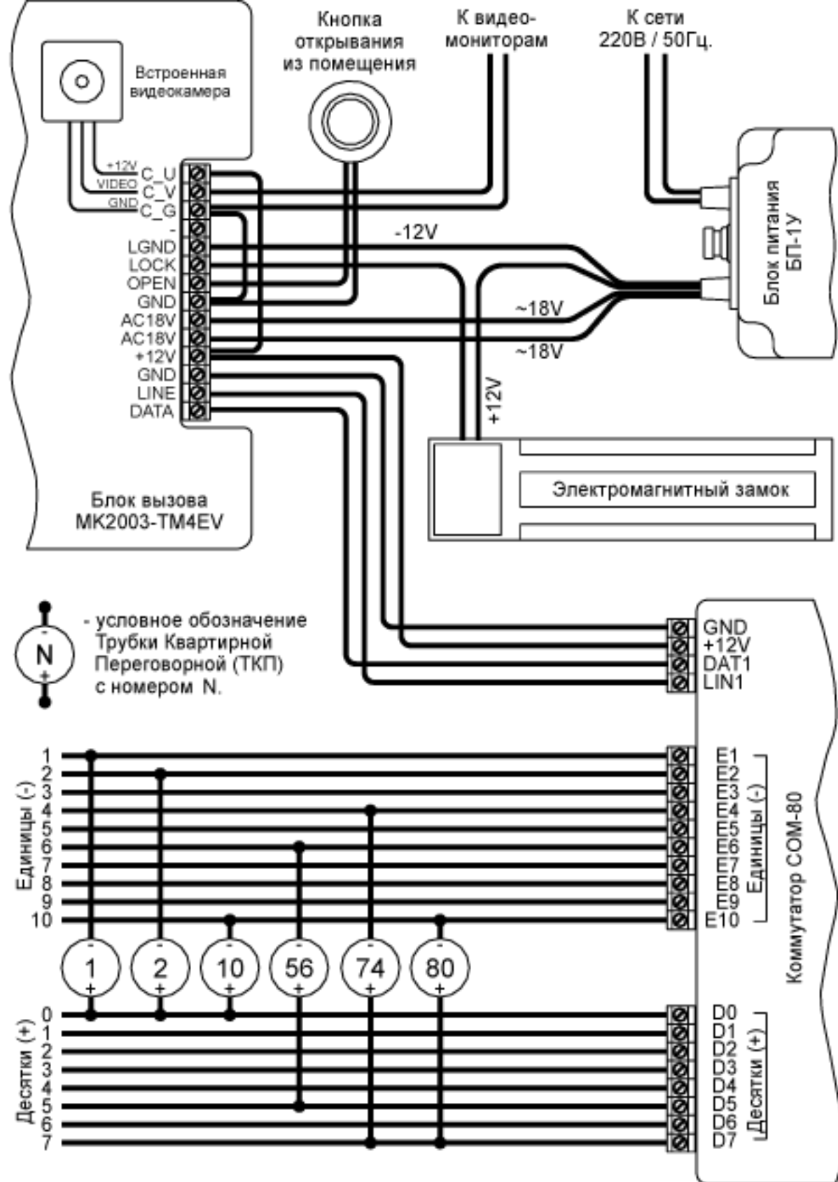
Пример монтажа блока вызова МК2003-ТМ4ЕV с коммутатором COM-80.
